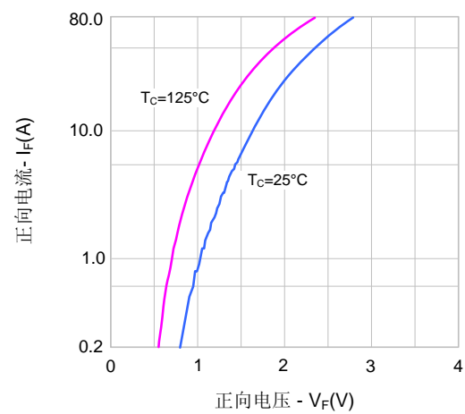
图12. 正向特性
