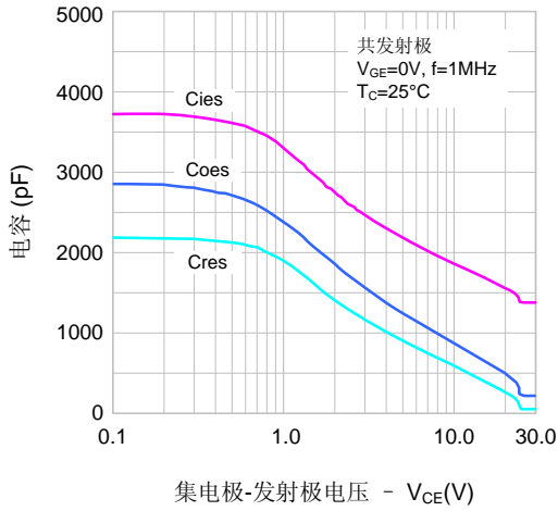
图7. 电容特性
